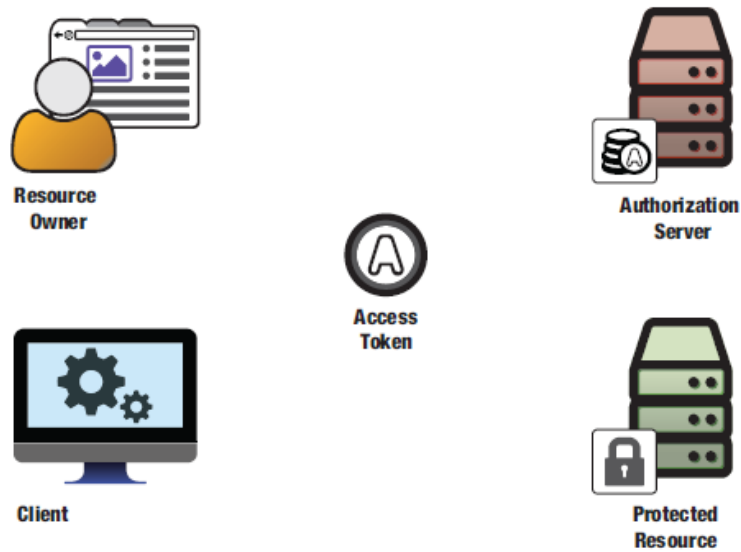
Abbildung 1 Die Rollen bei OAuth 2.0
