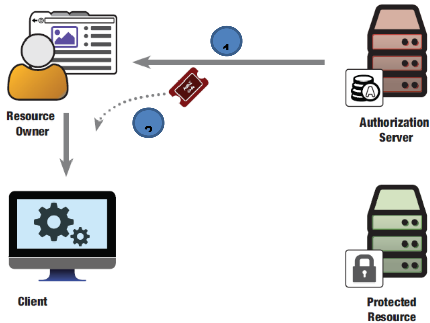
Abbildung 3 Der Authorization server übermittelt einen Authorization Code an den Client
