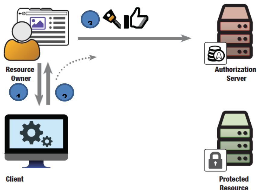
Abbildung 2 Der Client leitet den Resource owner zur Authentifizierung und Genehmigung an den Authorization server weiter
