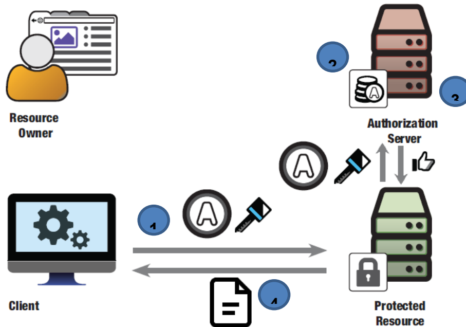
Abbildung 4 Verwendung eines Access Token, um auf eine mit OAuth geschützte Ressource zuzugreifen
